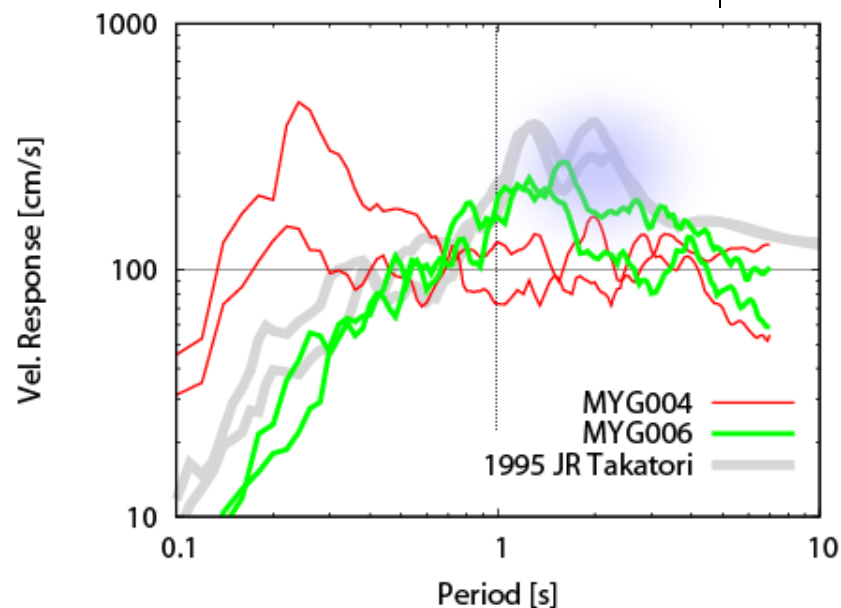
速度応答スペクトル
