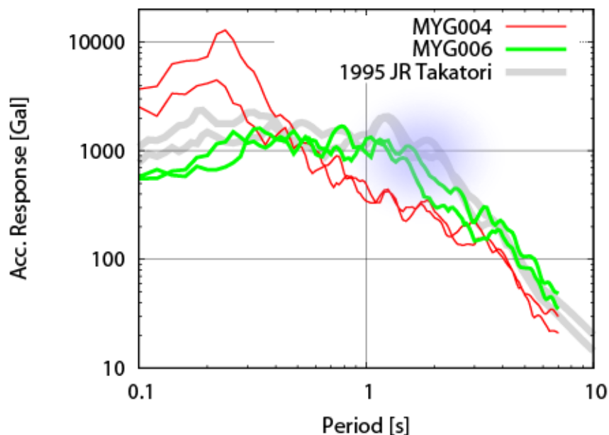
加速度応答スペクトル
